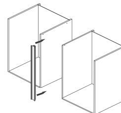
2. Вертикальная профиль-ручка GOLA средняя арт. 80/G1.5AL
