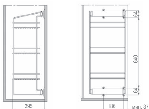
Присадочные размеры
