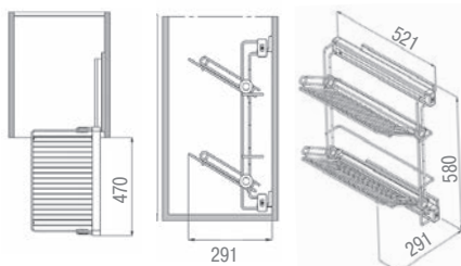
Габаритные размеры
