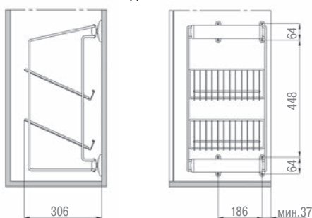
Присадочные размеры
