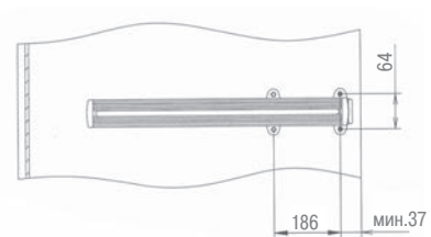
Присадочные размеры для установки держателя
