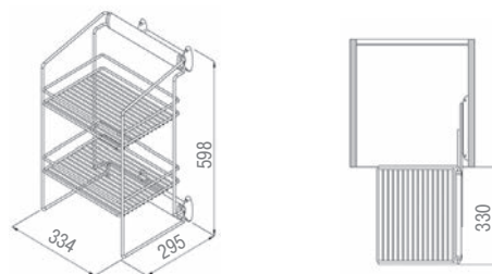
Присадочные размеры
