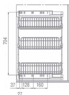
Присадочные размеры
