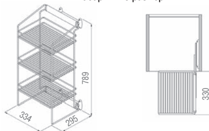
Присадочные размеры
