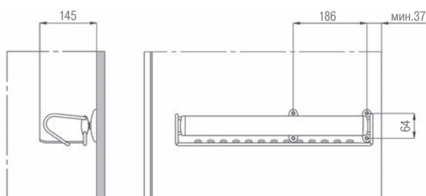
Присадочные размеры для установки держателя
