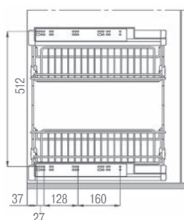
Присадочные размеры
