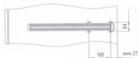
Присадочные размеры для установки держателя
