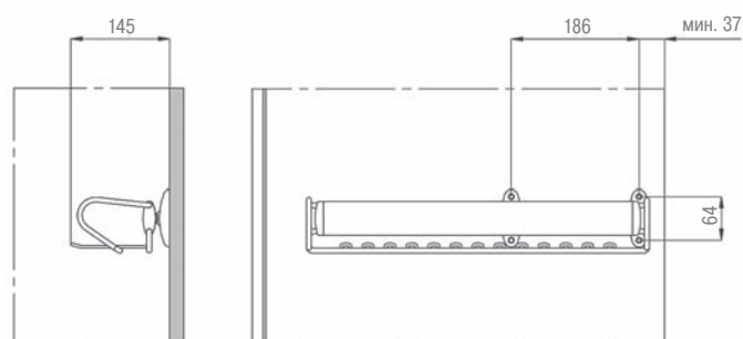
Присадочные размеры для установки держателя
