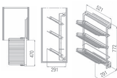
Габаритные размеры
