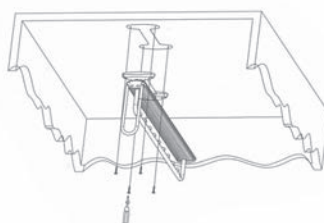
Присадочные размеры для установки держателя
