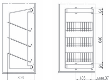
Присадочные размеры
