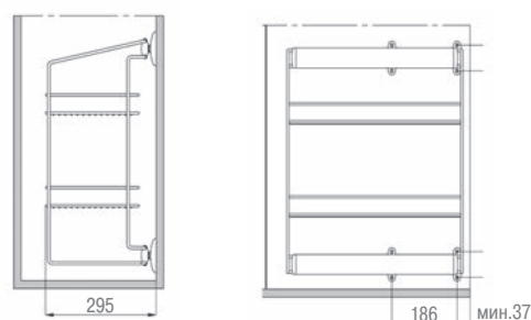
Присадочные размеры
