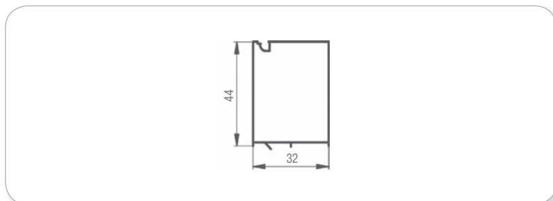
Заглушка скольжения для профиля MR 270
