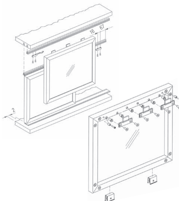
Схема установки механизма раздвижения для двойной двери
