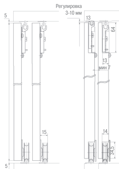
Габаритные размеры системы FAST
