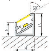
Габаритные размеры
