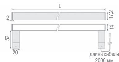
Установка светильника
