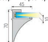
Габаритные размеры
