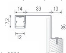
Габаритные размеры
