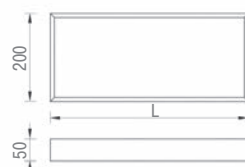
Габаритные размеры
