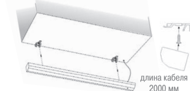
Установка светильника
