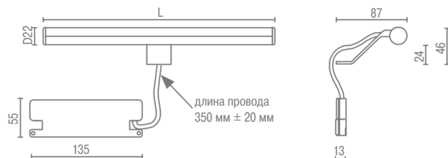
Габаритные размеры
