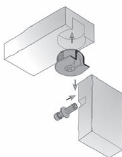
Стяжка эксцентриковая для полок
