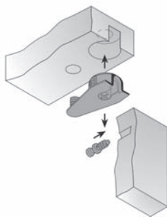
Стяжка эксцентриковая для полок, усиленная
