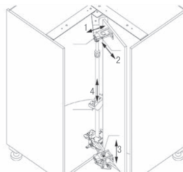
4. Регулировка полки по высоте
