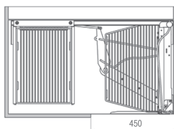
Габаритные размеры
