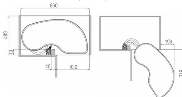
«Правая» версия
