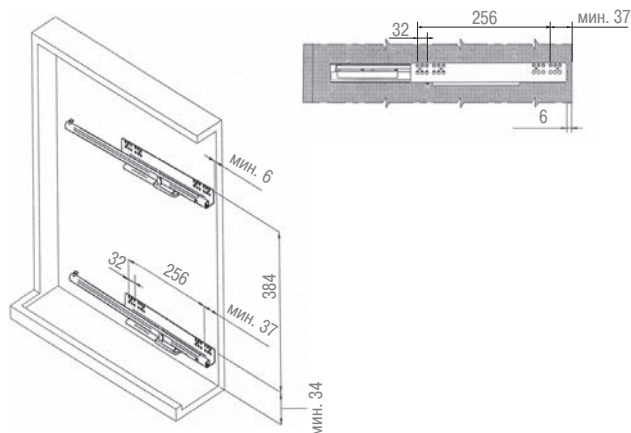
Присадочные размеры для установки направляющих
