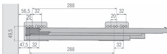
Присадочные размеры для установки направляющих NOVA PRO для решетчатой емкости GALAXY
