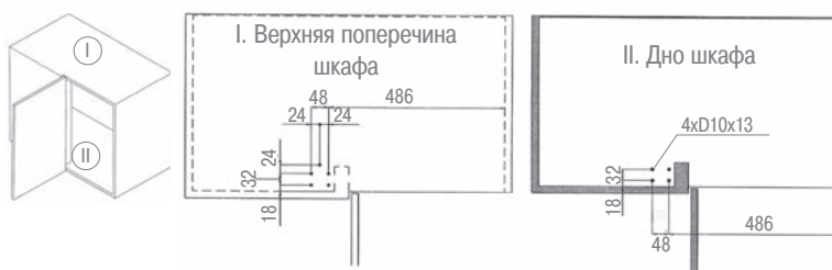
Присадочные размеры для крепления механизма
