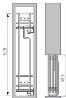
Габаритные размеры
