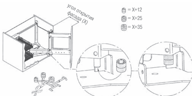
Изменение угла открытия фасада
