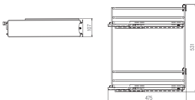
Габаритные размеры
