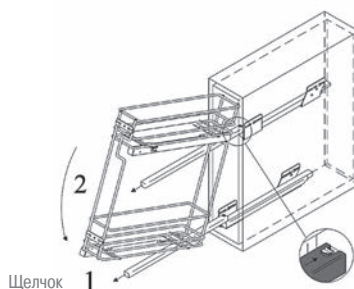
Установка направляющих и корзины
