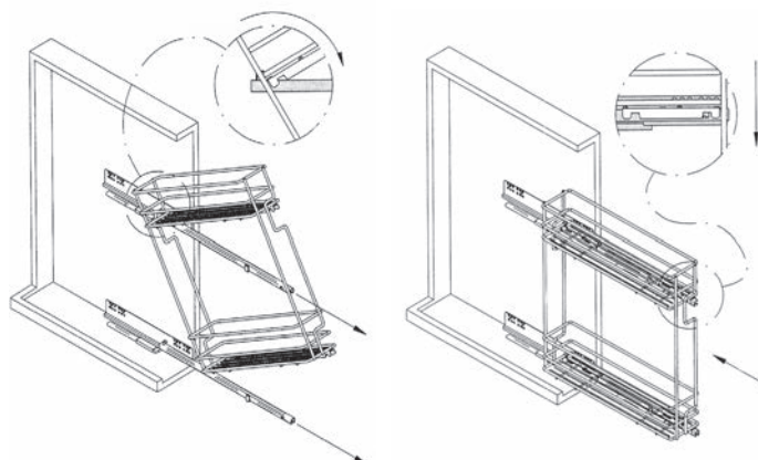
Установка корзины на направляющие
